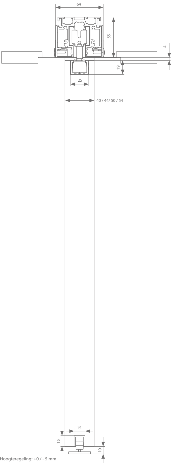
Voor systeemplafond (1+2)
