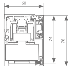
Muurbevestiging 40 mm
