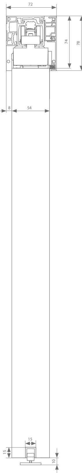
Muurbevestiging 54 mm
