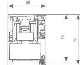
Muurbevestiging 44 mm
