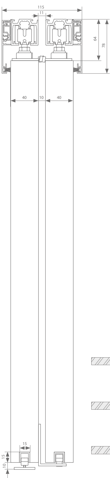
Parallelle plafondbevestiging 2
