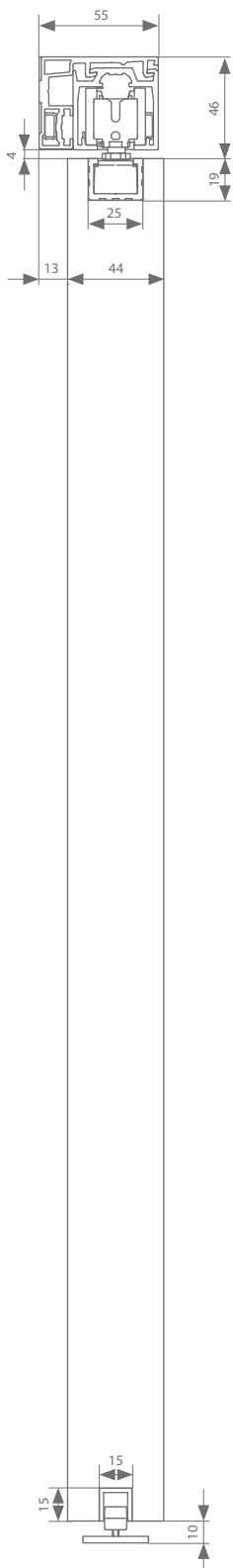
Muurbevestiging 44 mm
