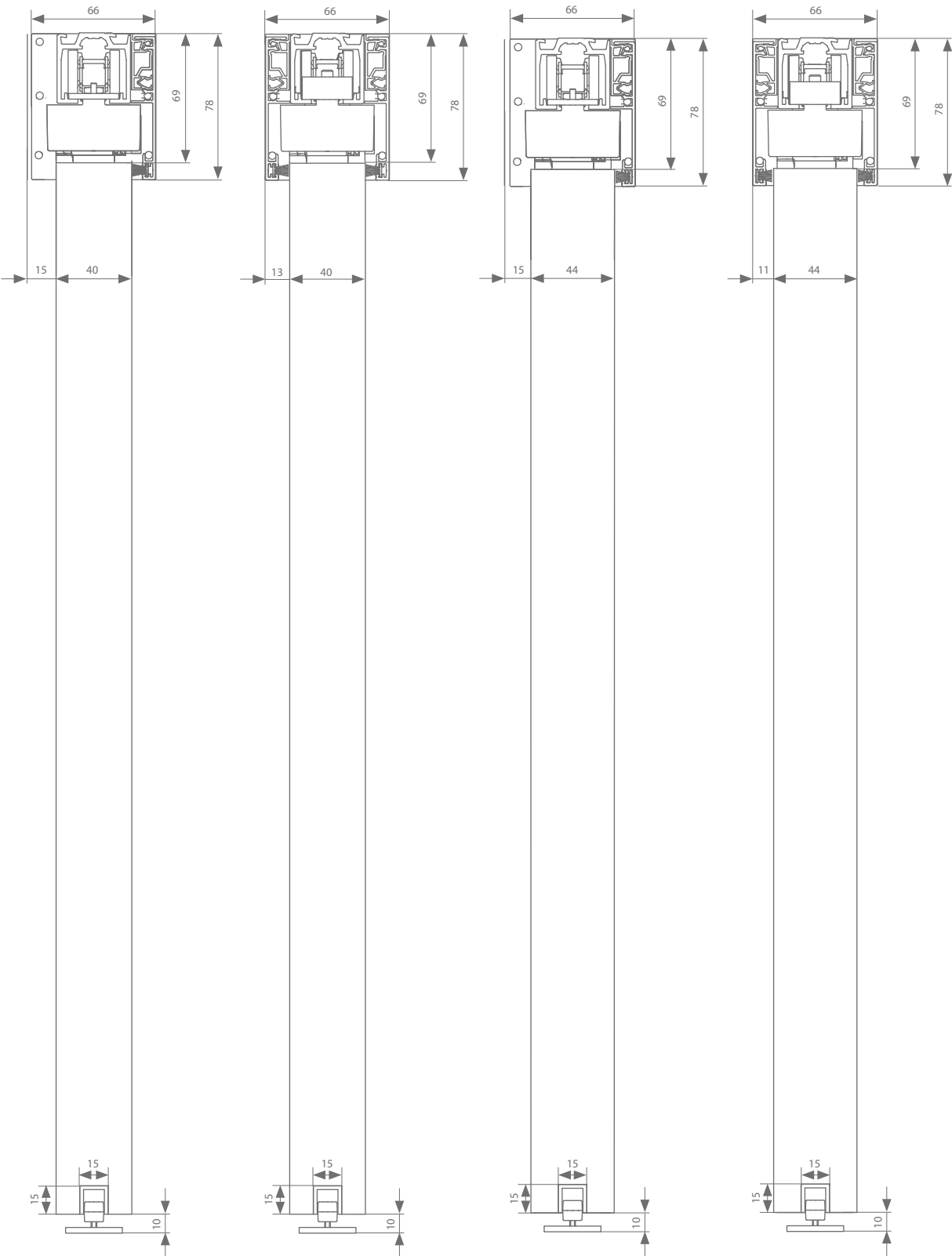
Plafondbevestiging 40 mm
