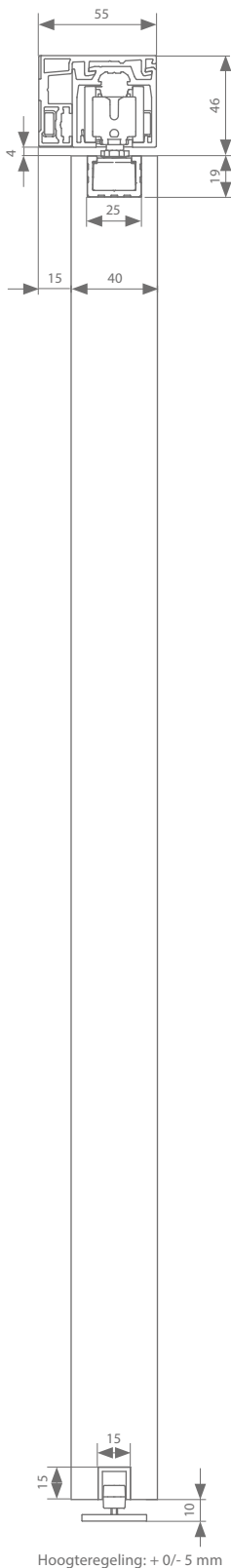
Muurbevestiging 40 mm
