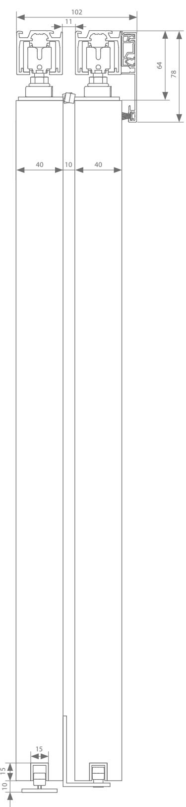
Parallelle plafondbevestiging 1
