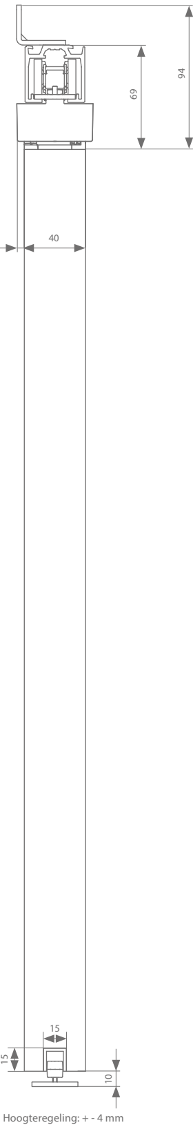
Muurbevestiging 40 mm
