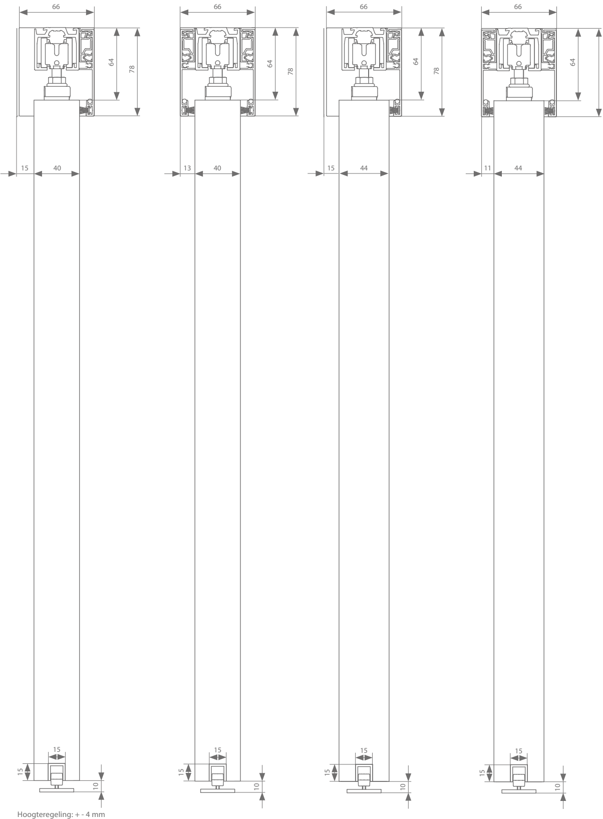
Plafondbevestiging 40 mm
