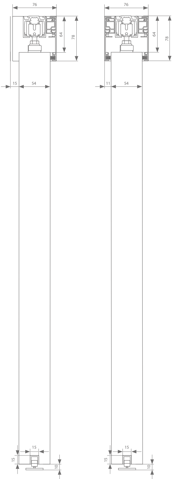
Plafondbevestiging 54 mm
