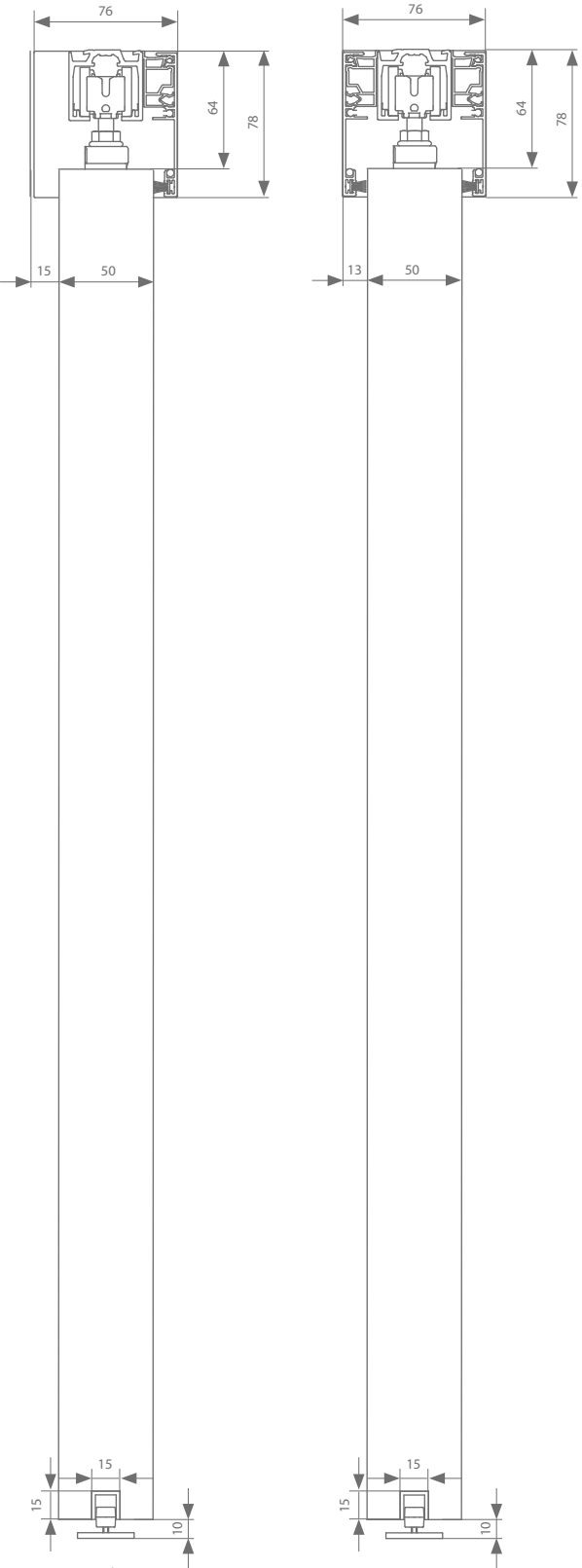
Plafondbevestiging 50 mm
