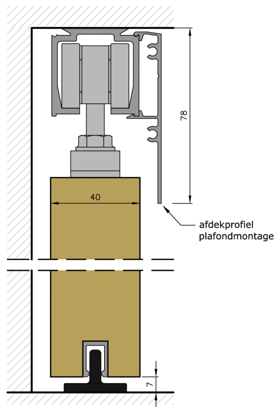
plafondbevestiging met afdekprofiel plafondmontage
