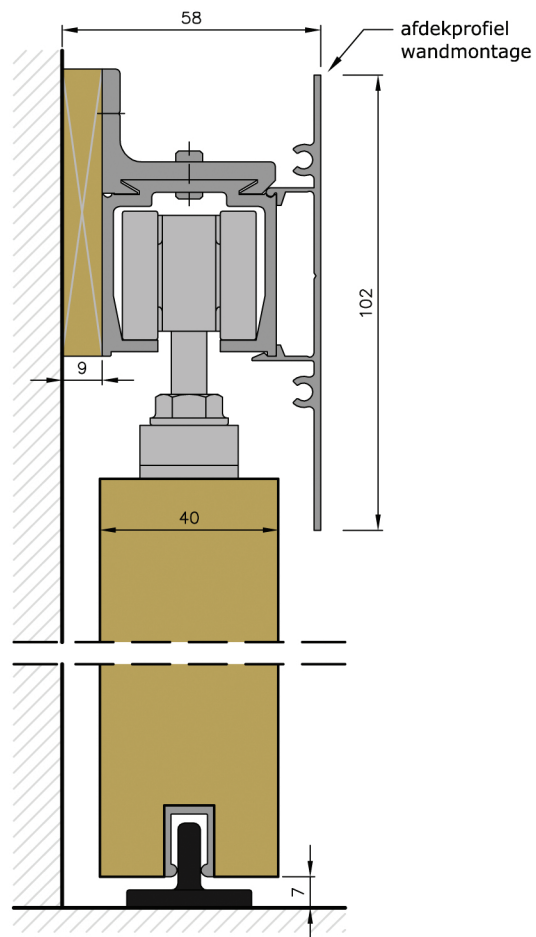
wandbevestiging met afdekprofiel wandmontage
