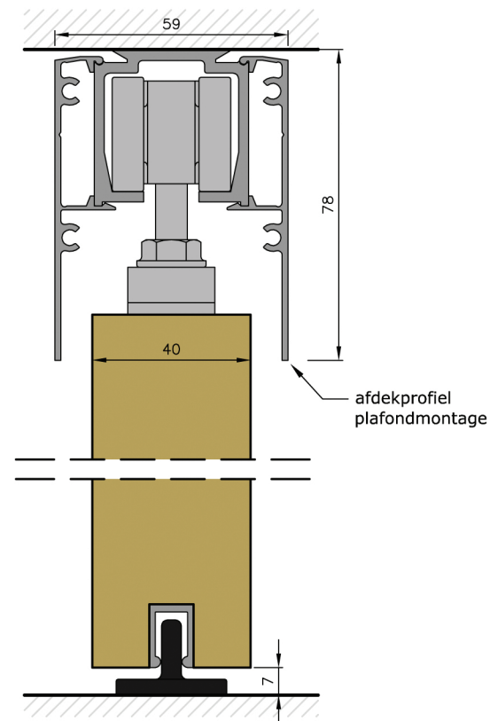
plafondbevestiging met afdekprofiel plafondmontage aan twee kanten
